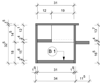
Schnitt 2 - 2
