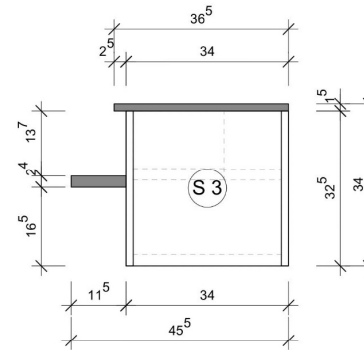
Seitenansicht
