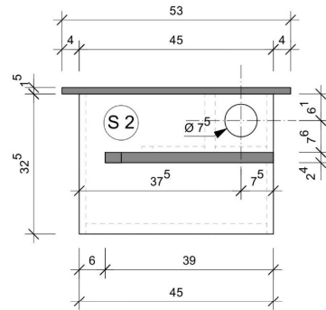
Seitenansicht
