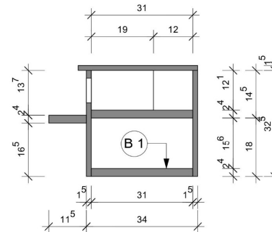
Schnitt 3 - 3
