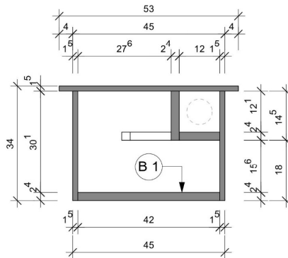
Schnitt 1 - 1
